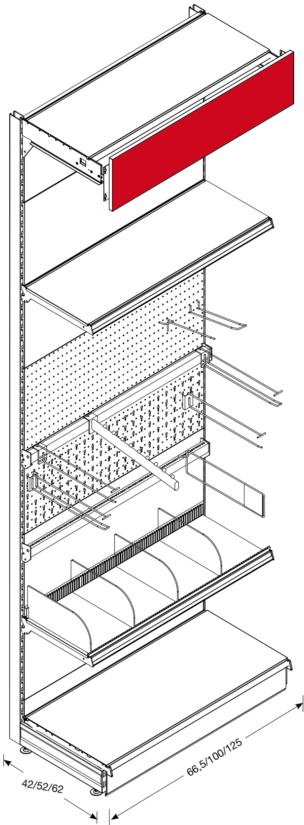
NY.01 SCAFFALE SINGOLO SINGLE SHELF
